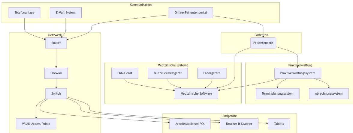
Figure 34.1: Beispiel IT-Architektur
